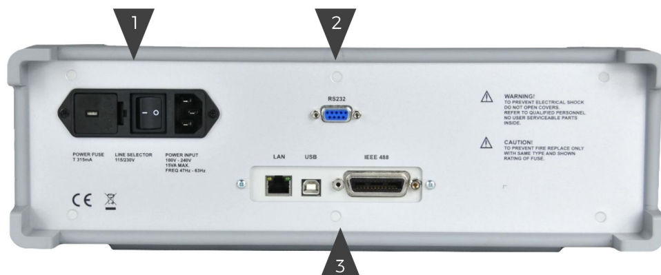
Obr. 3 Zadní panel
