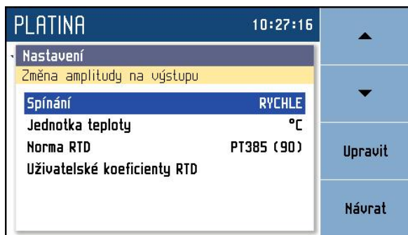
Obr. 7 Nastavení parametrů
