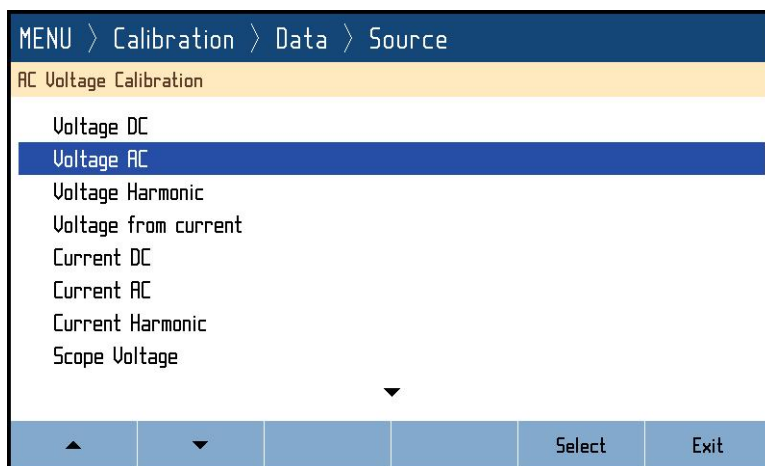
Obr. 49 Kalibrační menu
