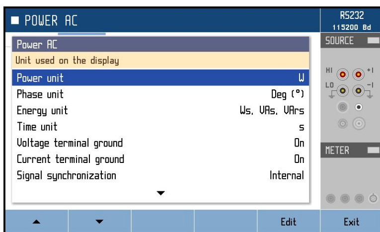
Obr. 31 Nabídka Power SETUP
