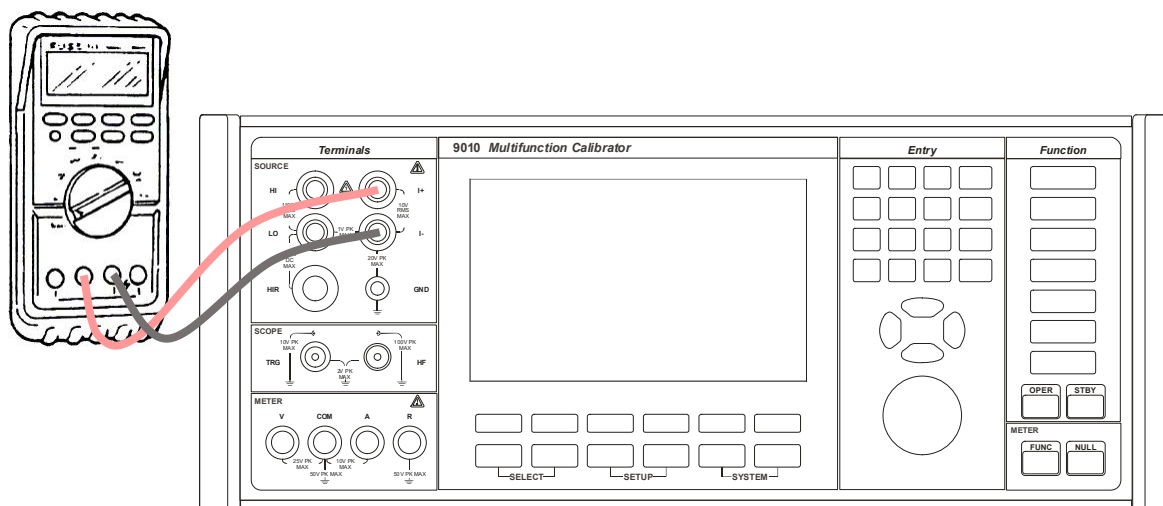
Obr. 20 Kalibrace ampérmetru
