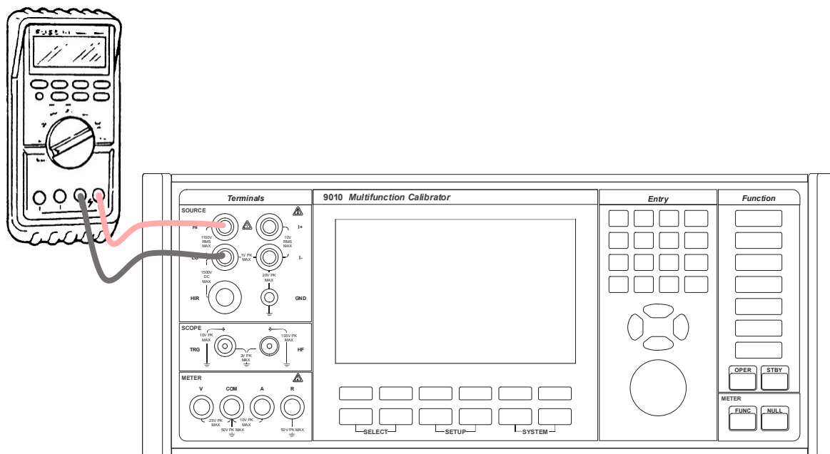
Obr. 15 Kalibrace voltmetru
