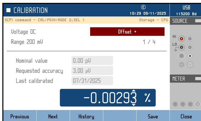
Obr. 50 Přímá kalibrace daného bodu
