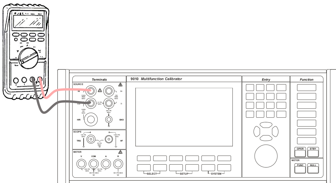
Obr. 22 Kalibrace odporu ve dvousvorkovém zapojení
