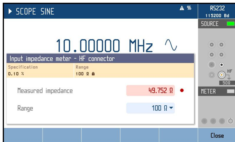
Obr. 37 Měření vstupní impedance - SCO option
