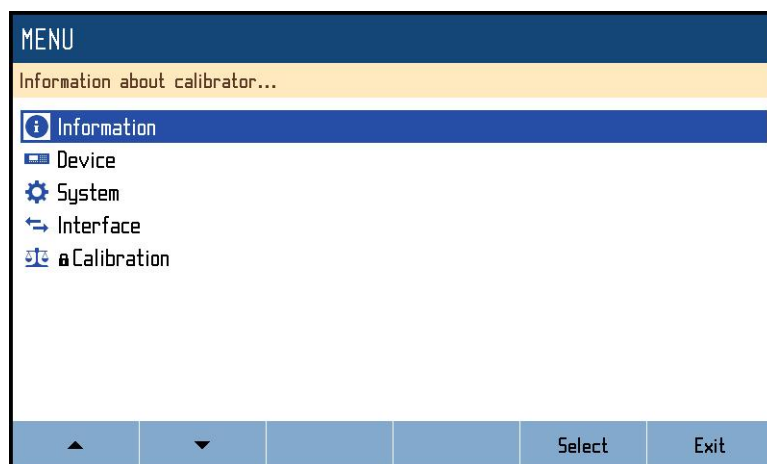
Obr. 10 Hlaní menu
