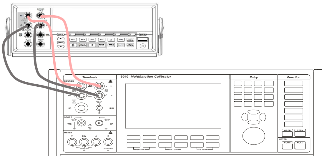
Obr. 27 Kalibrace měřidla výkonu
