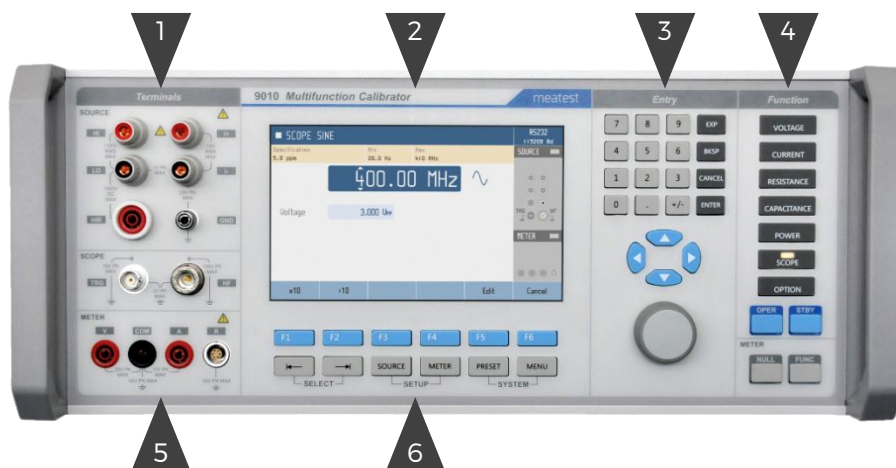
Obr. 1 Přední panel
