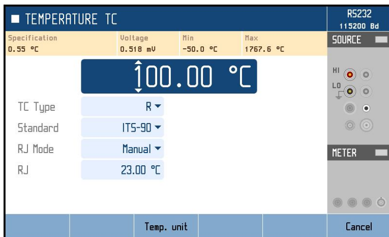
Obr. 40 Simulace termočlánků TC
