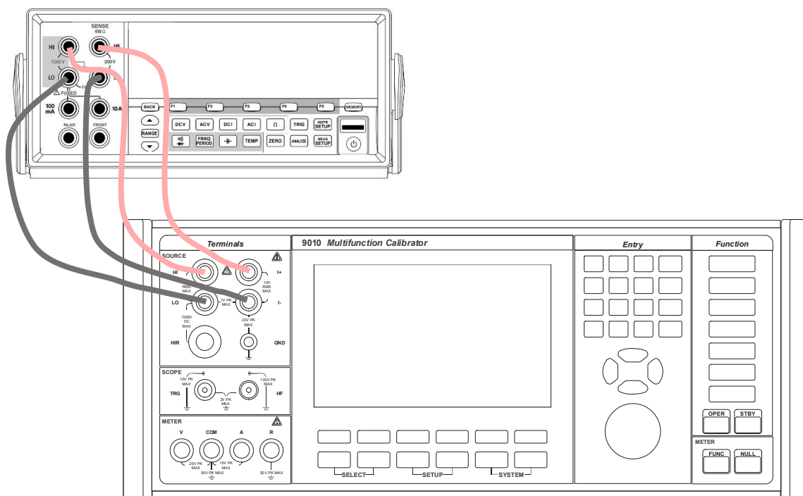
Obr. 23 Kalibrace odporu ve čtyřsvorkovém zapojení
