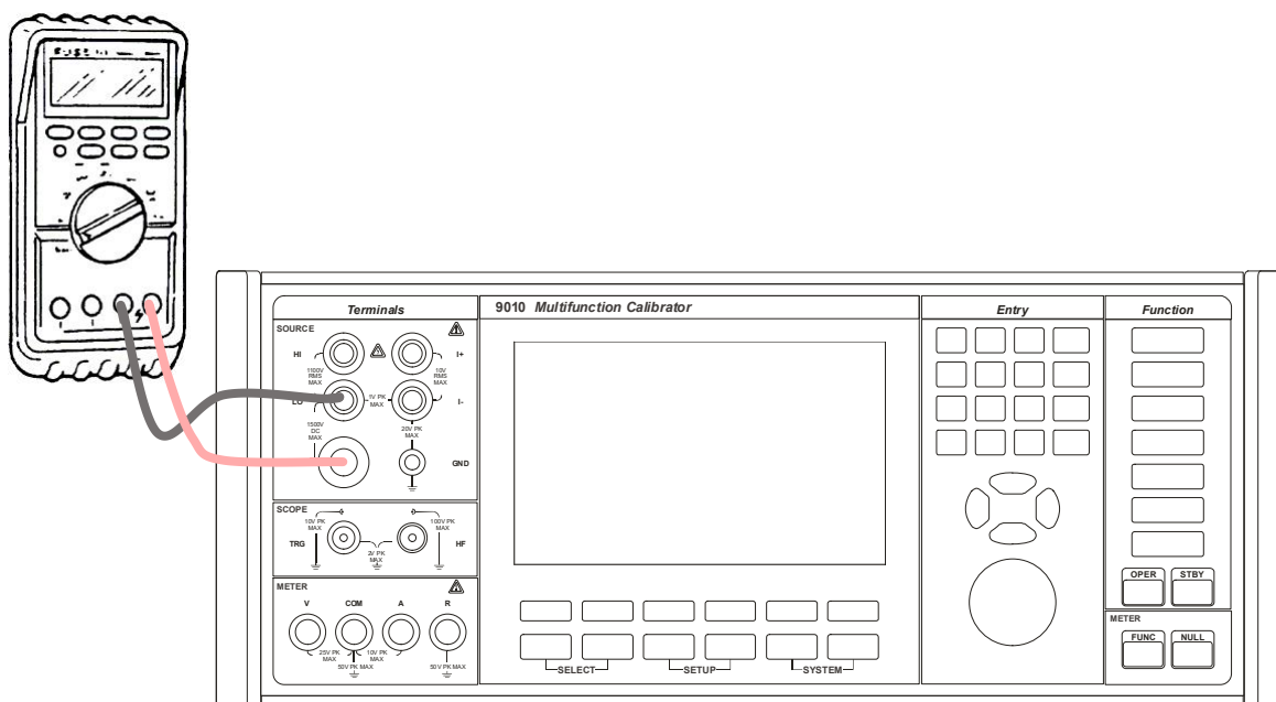
Obr. 24 Kalibrace odporu vysokých hodnot
