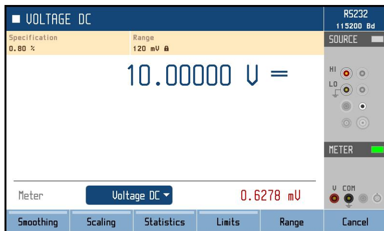
Obr. 42 Procesní multimetr
