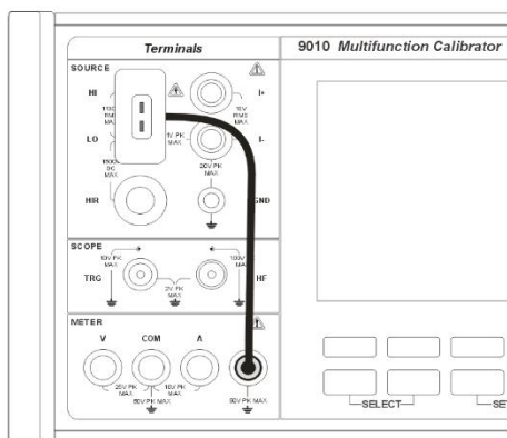
Obr. 41 Automatická kompenzace studeného konce TC s pomocí adapter-Adapter 91
