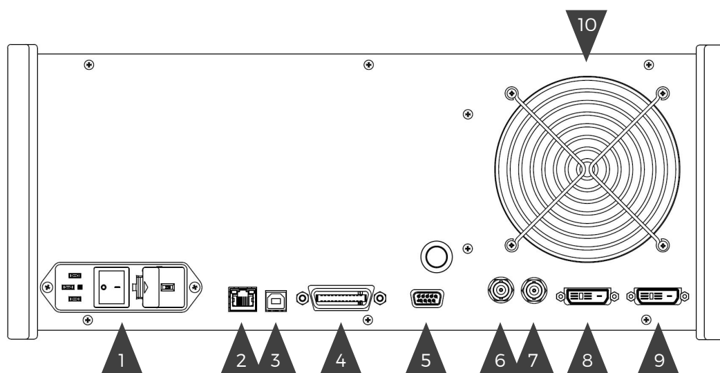
Obr. 6 Zadní panel
