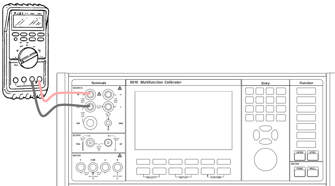
Obr. 25 Kalibrace kapacity
