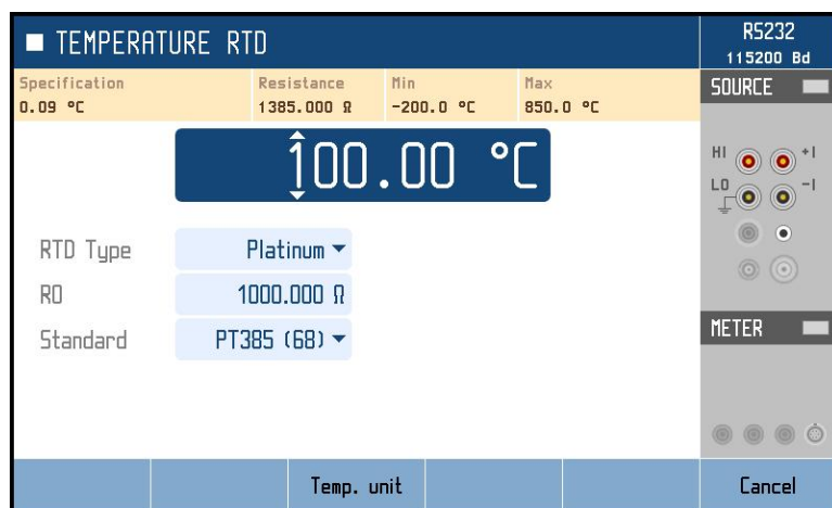
Obr. 39 Simulace odporových snímačů teploty RTD
