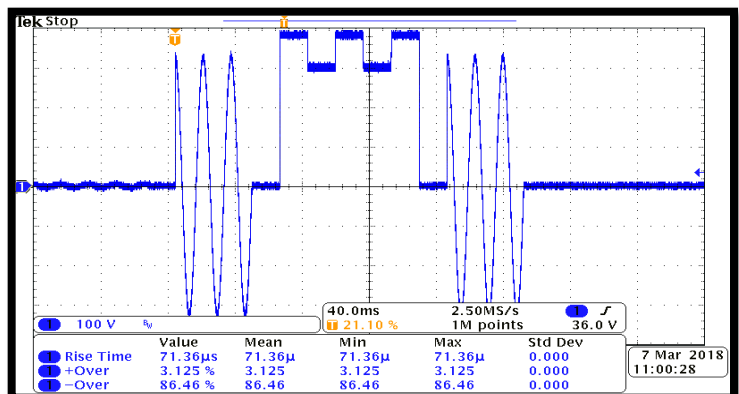
Actual output voltage waveform
